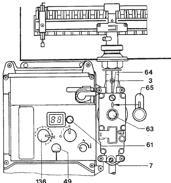
Obr. 37 Plynová armatura CE 426 pro zemní plyn a propan-butan (butan)
