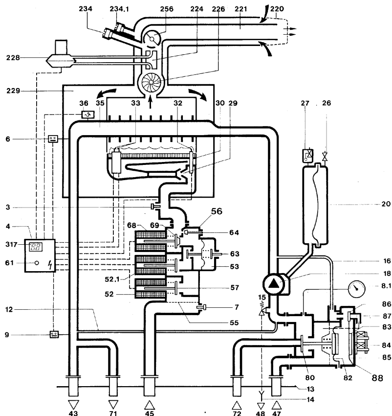
Obr.3 CERASTAR ZR přestavěn na ZSR s příslušenstvím 442 (zemní plyn a propan - butan)
